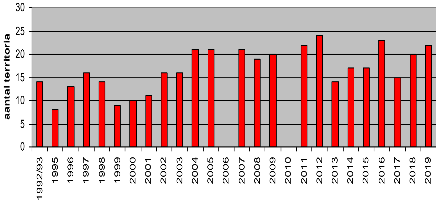
roodborsttapuit bmp-plots groote peel 1992/93-2019
