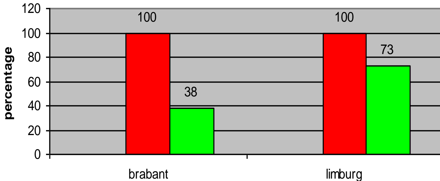
procentuele afname brabant en limburg 2018 (rood) - 2019 (2018 = 100%)
